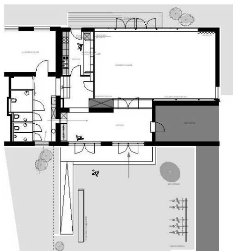
Grundriss Gemeindesaal Weiler&Köhle
